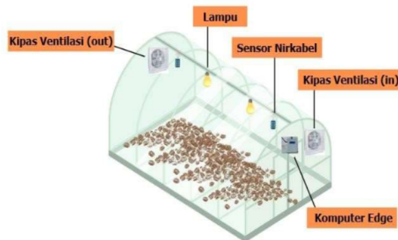
Gambar 2. Skema Greenhouse Terintegrasi IoT
