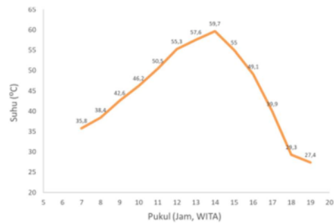
Gambar 6. Grafik Suhu Greenhouse Sebelum Terintegrasi IoT
