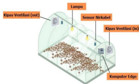
Gambar 4. Skema Greenhouse Terintegrasi IoT
