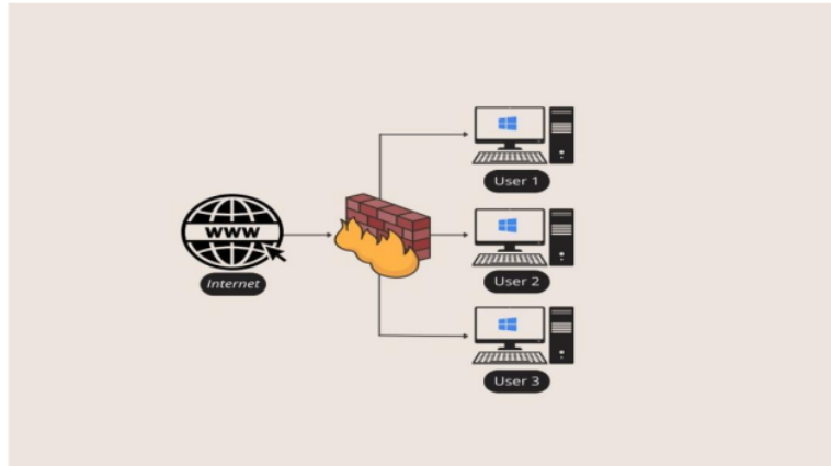
Gambar 4.5 ilustrasi firewall
