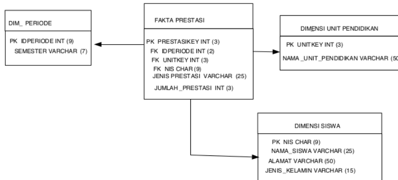
Gambar 6. Star skema fakta prestasi
