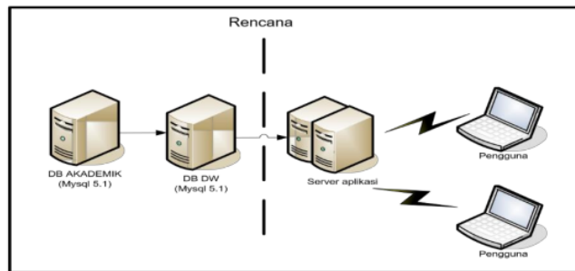
Gambar 4. Arsitektur fisik data warehouse
