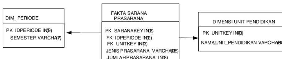
Gambar 5. Star skema fakta sarana prasarana
