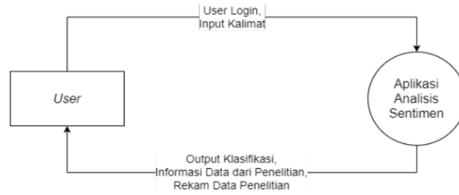
Gambar 3. Diagram Konteks
