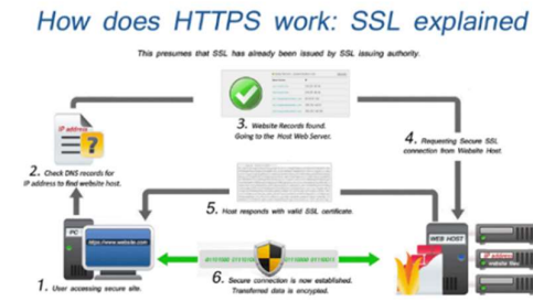
Gambar. 7. Cara kerja SSL/TLS
