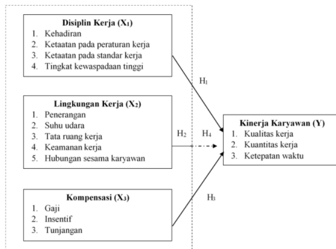
Gambar 2.1 Kerangka Konseptual
