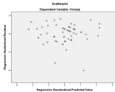
Gambar 1. Uji Heteroskedastisitas
