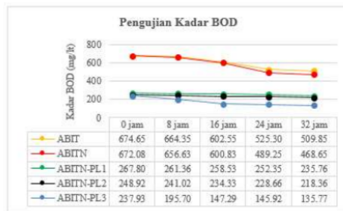
Gambar 4.2. Grafik Perubahan Kadar BOD
