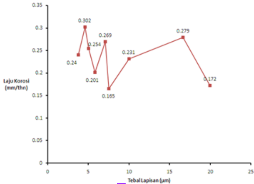
15 Gambar 4.3 (Grafik ketebalan lapisan vs laju korosi)
