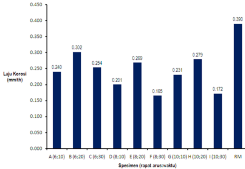
Gambar 4.2 Grafik laju korosi pada setiap sampel
