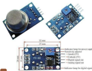
Gambar 2.6 Sensor MQ135
