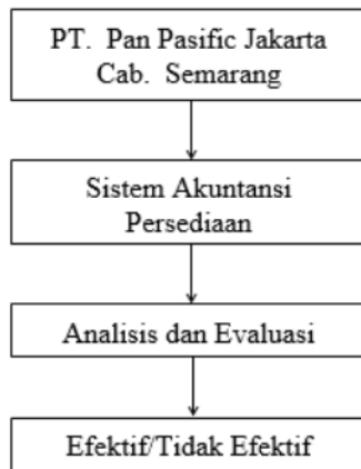
Gambar 2.3 Kerangka Pikir
