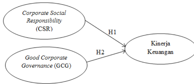
Gambar 1. Kerangka Penelitian
